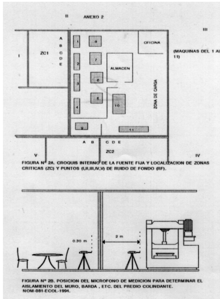
FIGURA No. 2B. POSICION DEL MICROFONO DE MEDICION PARA DETERMINAR EL AISLAMIENTO DEL MURO, BARRA, ETC. DEL PREDIO COLINDANTE.
